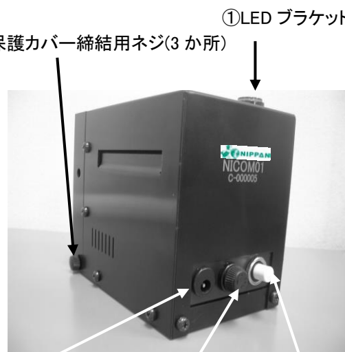
④ACアダプタープラグロ ③ヒューズホルダー ②電源スイッチ
