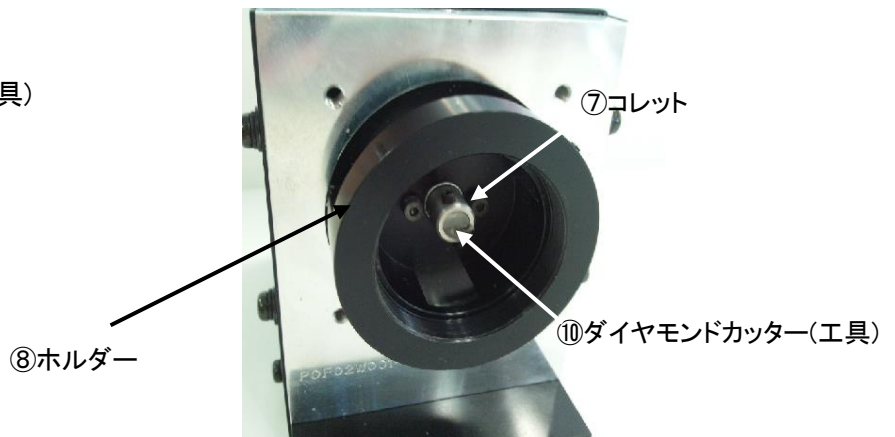
[前面保護カバーとアタッチメントを取り外した状態]
